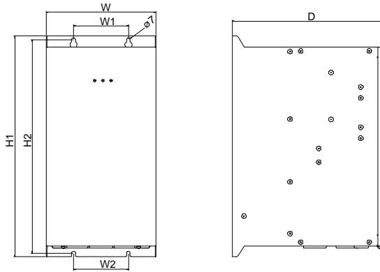
图 3-3 320A-400A 尺寸图
