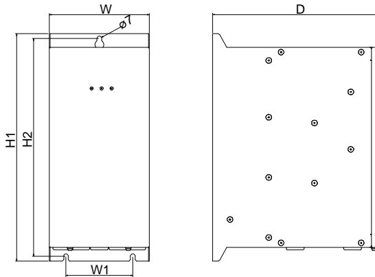
图 3-2 110A-220A 尺寸图
