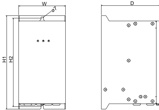
图 3-1 60A 尺寸图
