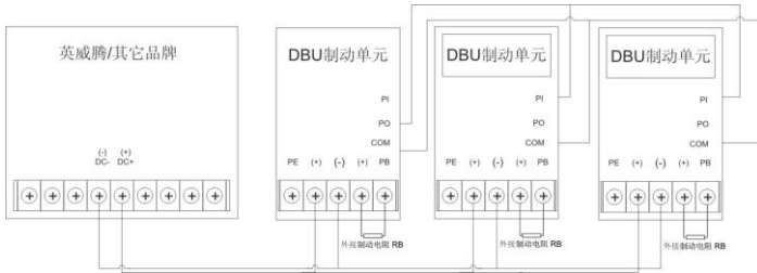
图 6-1 制动单元并联运行与变频器连线图
