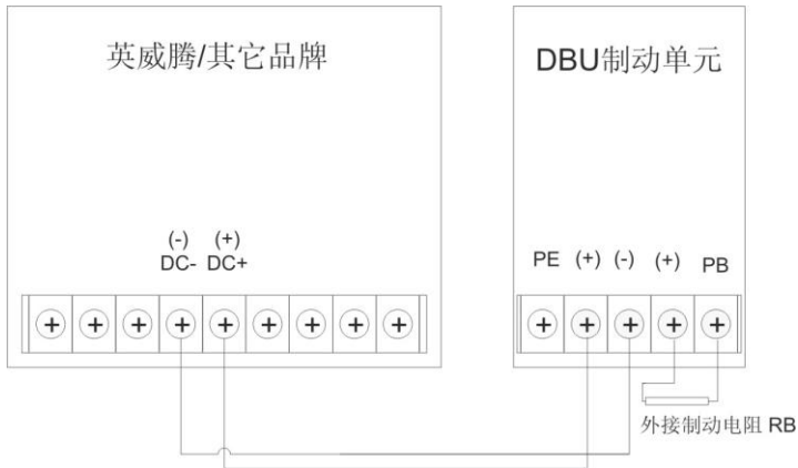
图 5-1 制动单元与变频器主回路接线图
