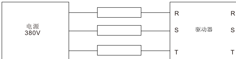
图 11.1 380V 驱动装置充电电路示例
