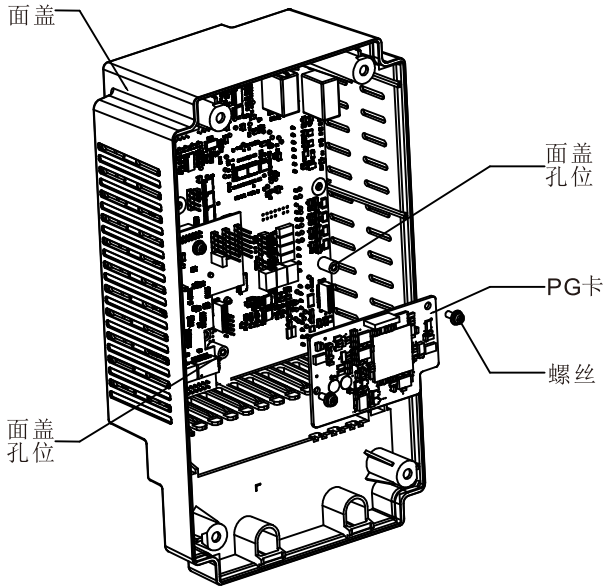
图 A.2 编码器 PG 扩展卡安装图
