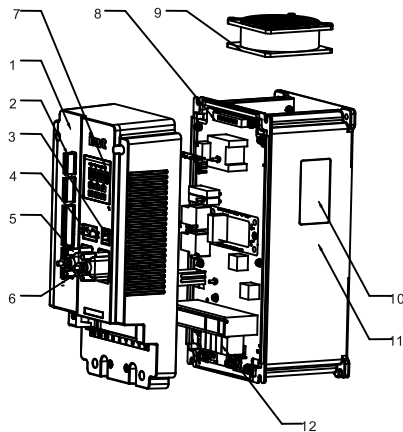
图 3.5 结构示意图
