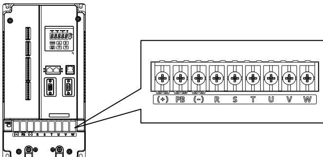
图 5.3 380V 7.5~15kW 主回路端子示意图
