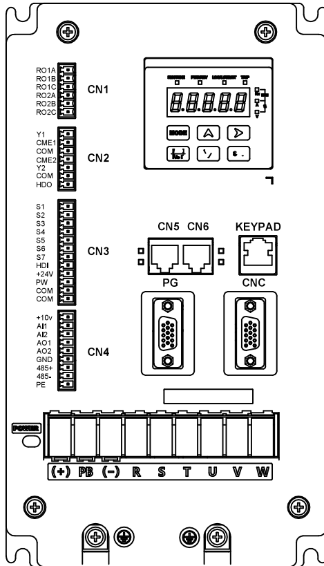
图 5.6 端子排列图
