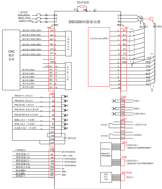
图 5.11 双路增量式编码器控制回路接线图
