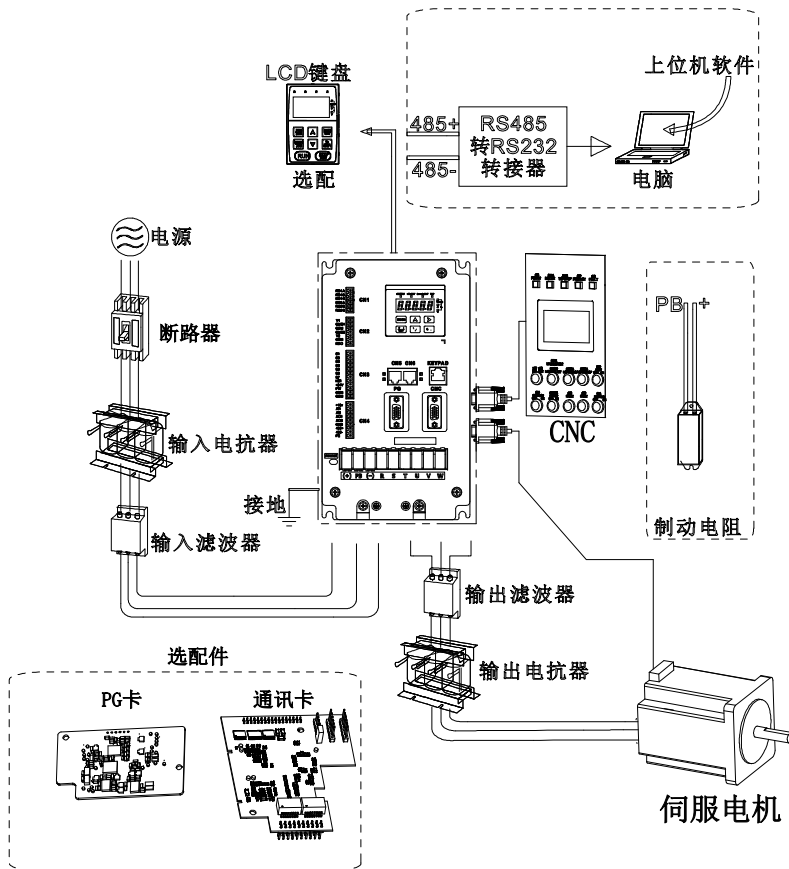
图 3.2 系统构成图
