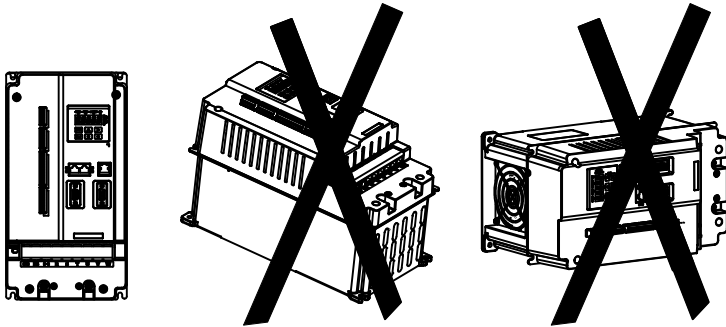
图 4.2 伺服主轴驱动器安装方向
