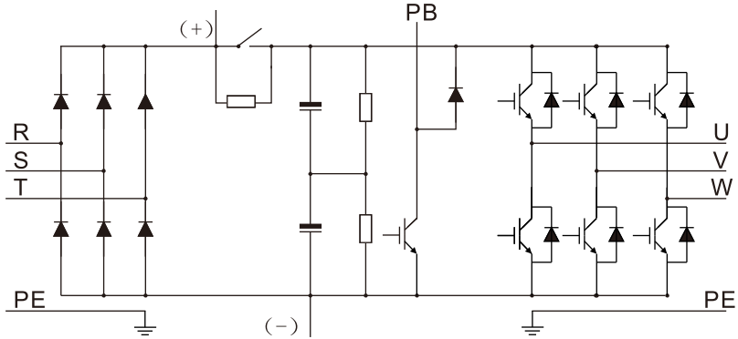
图 3.1 380V (2.2kW~15kW) 主回路简图
