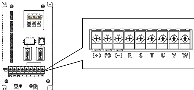
图 5.2 380V 2.2~5.5 kW 主回路端子示意图
