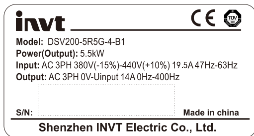
图 3.3 产品铭牌
