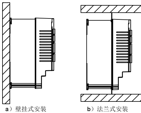
图 4.3 安装方式
