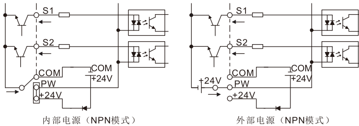
图 5.13 NPN 模式示意图
