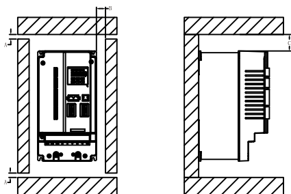
图 4.4 单台安装
