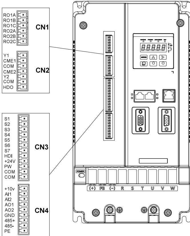
图 5.12 U 型短接位置示意图
