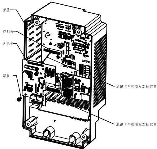
图 A.1 通讯选配卡安装图
