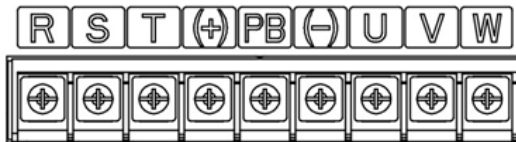
图 3.7 GD200A-02-045-4-A 主回路端子示意图
