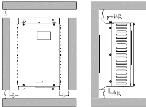
图 3.4 单台安装
