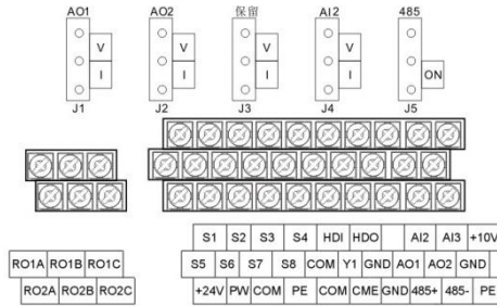
图 3.11 GD200A-02-045-4-A/GD200A-02-055-4-A 控制端子示意图
