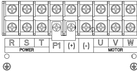
图 3.9 GD200A-02-055-4-A 主回路端子示意图
