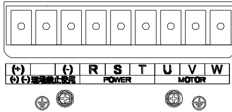
图 3.8 GD200A-02-022-4/GD200A-02-037-4 主回路端子示意图
