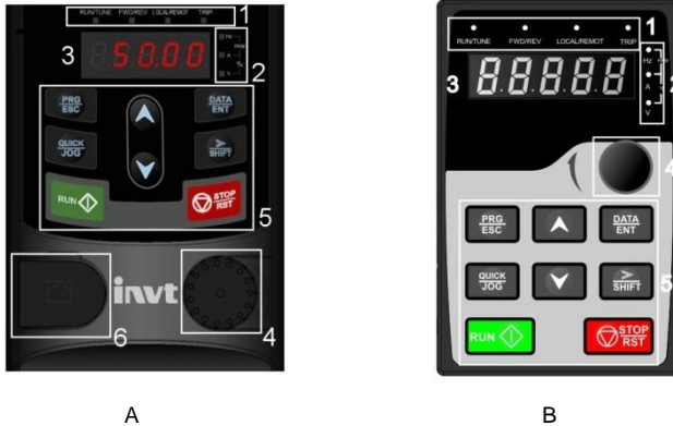
图 4.1 键盘示意图
