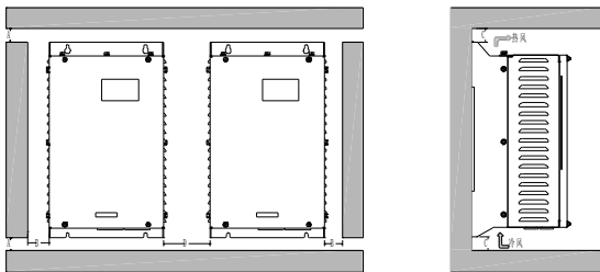
图 3.3 并行安装
