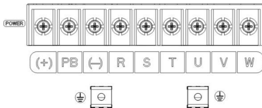
图 3.6 GD200A-02-022-4-A/GD200A-02-037-4-A 主回路端子示意图
