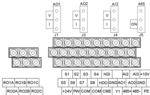
图 3.10 GD200A-02-022-4/GD200A-02-022-4-A/ GD200A-02-037-4/GD200A-02-037-4-A 控制端子示意图
