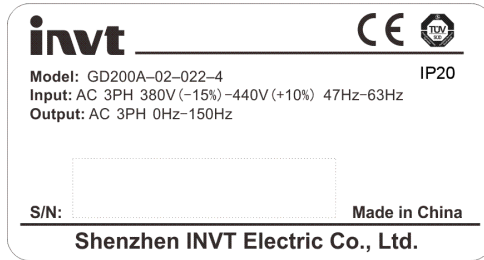
图 2.1 产品铭牌
