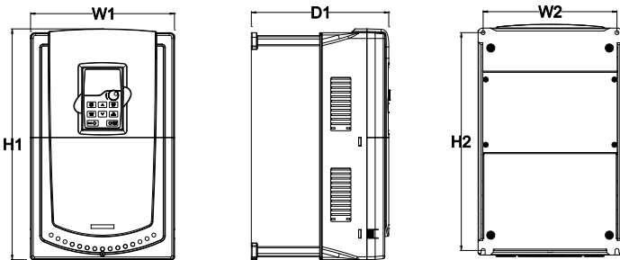
图 B.3 GD200A-02-045-4-A 壁挂安装示意图
