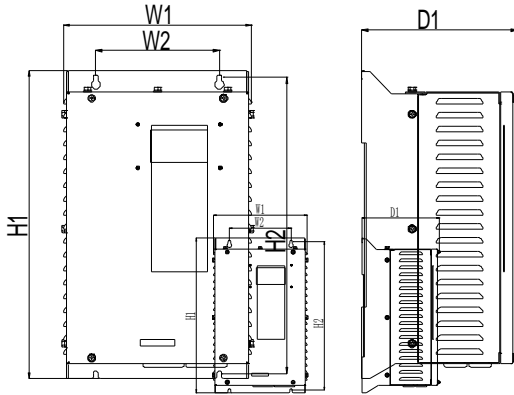
图 B.2 GD200A-02-022-4/GD200A-02-037-4 壁挂安装示意图
