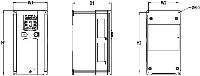
图 B.1 GD200A-02-022-4-A/GD200A-02-037-4-A 壁挂安装示意图
