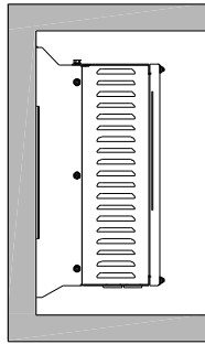
图 3.2 壁挂式安装
