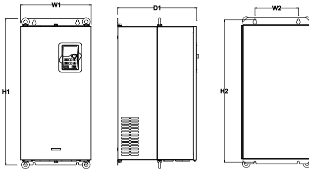
图 B.4 GD200A-02-055-4-A 壁挂安装示意图
