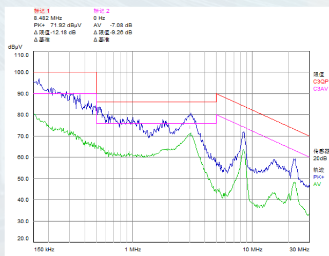
加滤波器后
