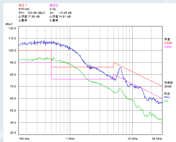
加滤波器前
