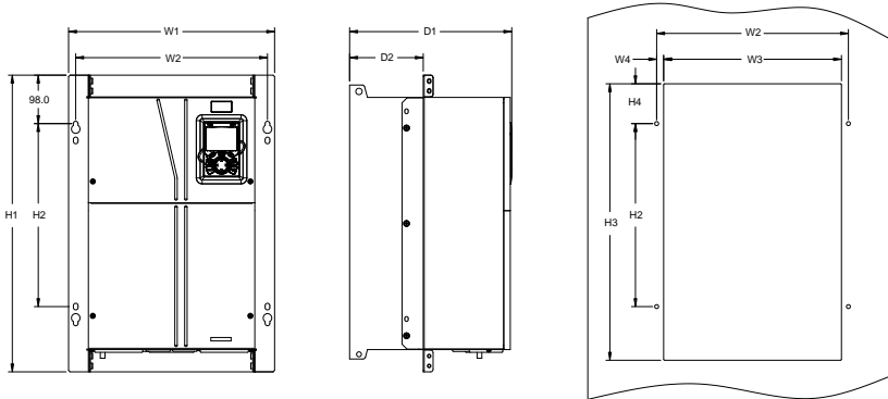
图 C-10 090G/110P~110G/132P 法兰安装示意图
