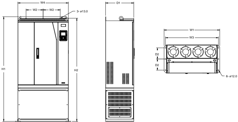
图 C-12 220G/250P~315G/355P 落地安装示意图
