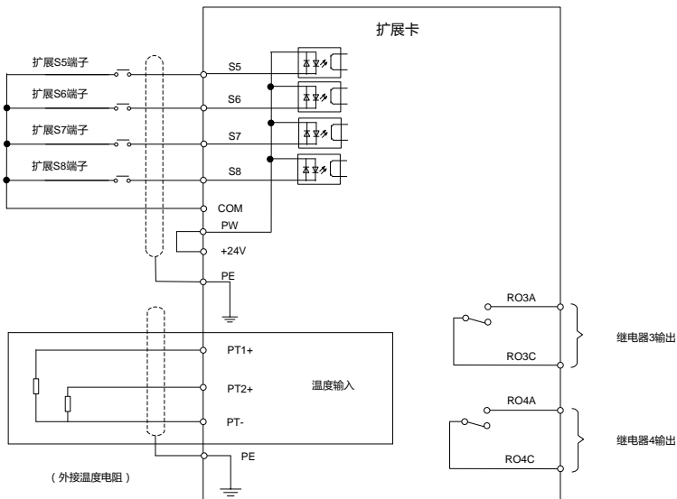
图 A-6 IO 扩展卡 2 控制回路接线图
