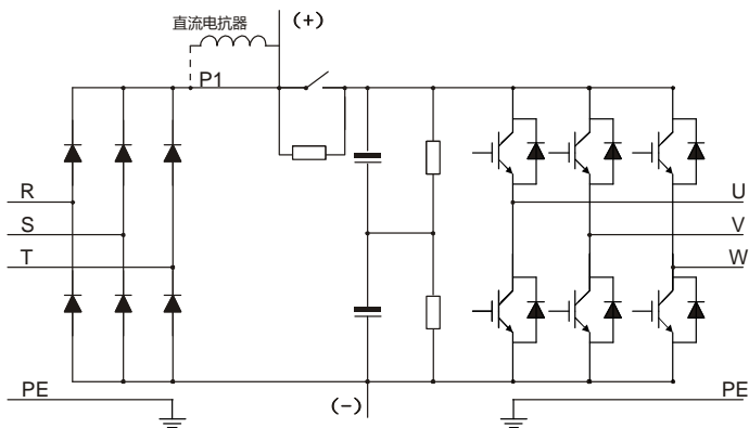
图 3-4 132G/160P 及以上主回路简图
