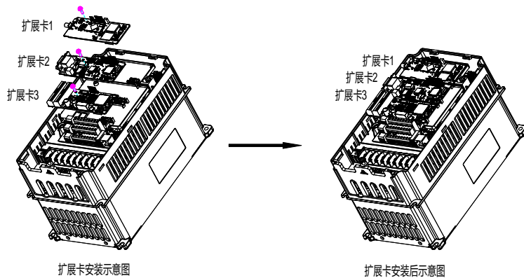
图 A-1 7R5G/011P (含) 以上机型效果图
