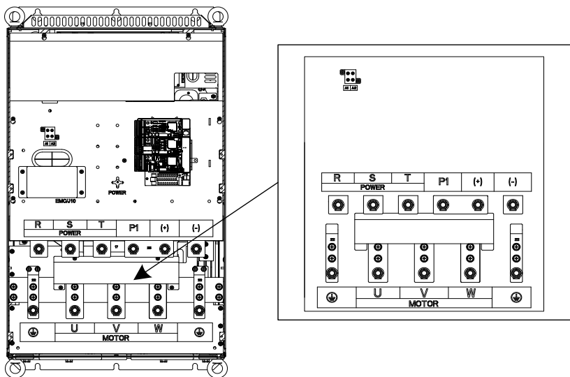
图 4-11 132G/160P~200G/220P 主回路端子示意图
