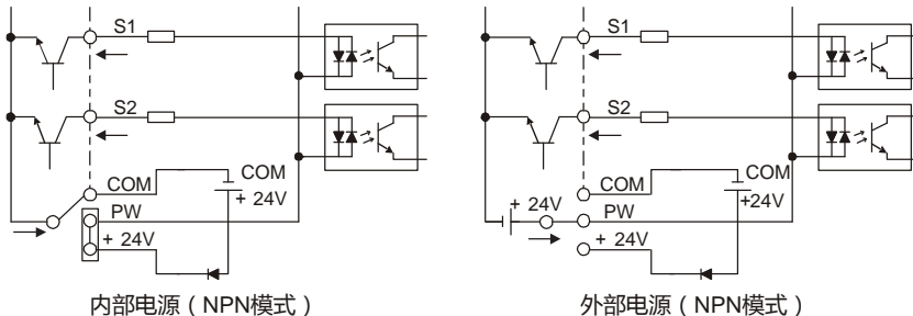
图 4-17 NPN 模式示意图
