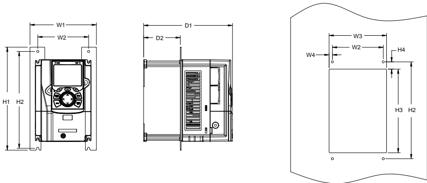
图 C-9 1R5G/2R2P~075G/090P 法兰安装示意图
