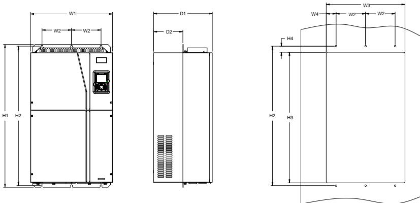
图 C-11 132G/160P~200G/220P 法兰安装示意图
