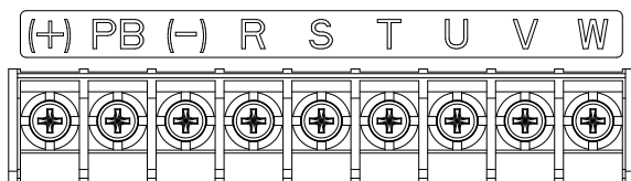
图 4-8 022G/030P（含）以下主回路端子示意图
