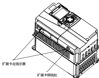
图 A-5 走线方式示意图
