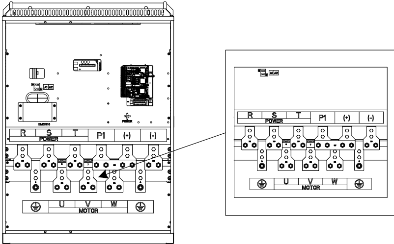
图 4-12 220G/250P~315G/355P 主回路端子示意图
