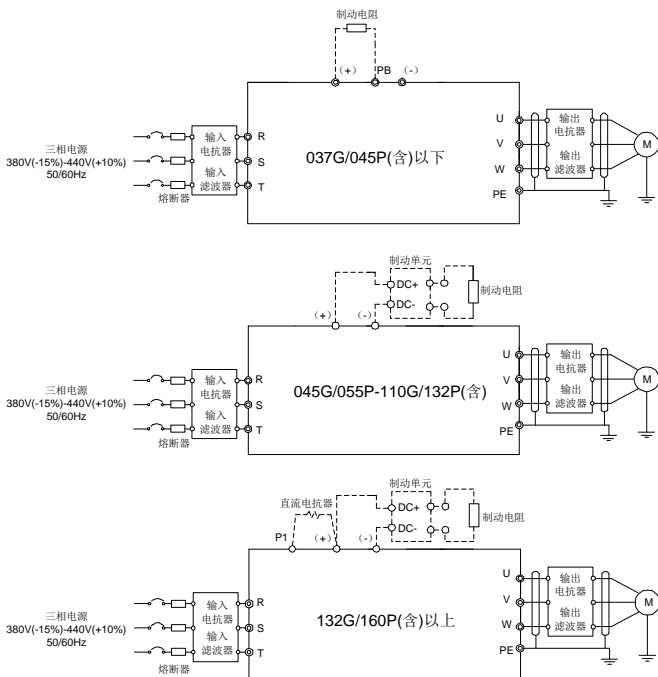
图 4-7 主回路接线图
