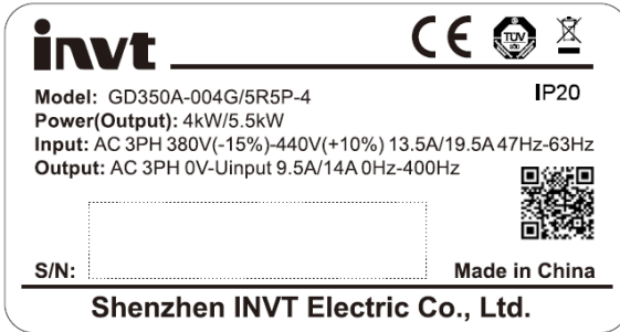
图 3-5 产品铭牌
