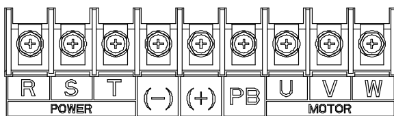
图 4-10 045G/055P-110G/0132P 主回路端子示意图（选配内置制动单元是启用 PB）
