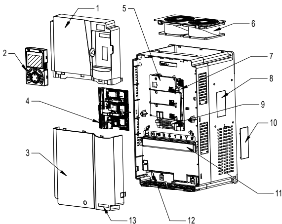
图 3-7 产品结构示意图
