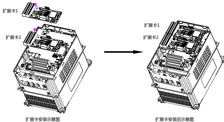
图 A-2 5R5G/7R5P (含) 以下机型效果图
