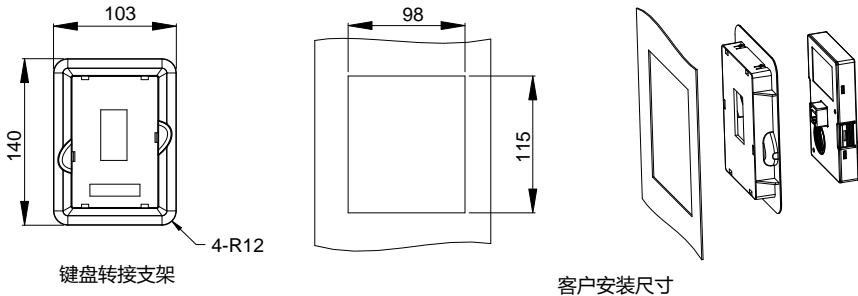
图 C-2 1R5G/2R2P-500G 键盘安装架 (选配) 图
