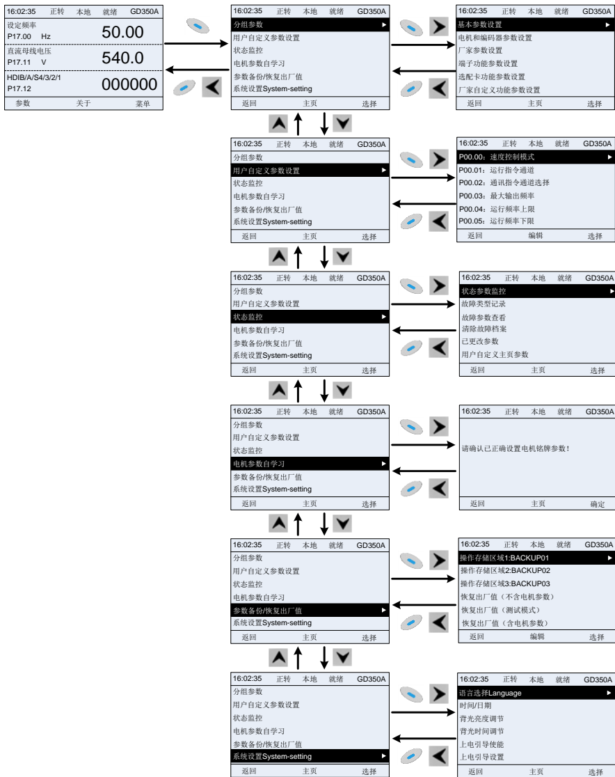
图 5-9 进入/退出各级菜单示意图 2
