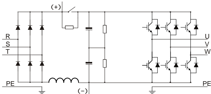
图 3-3 045G/055P~110G/132P 主回路简图
