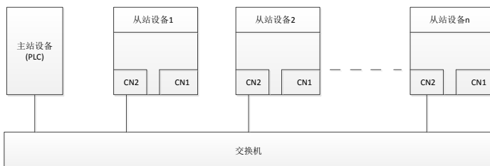
图 A-9 星型网络拓扑电气连接图
