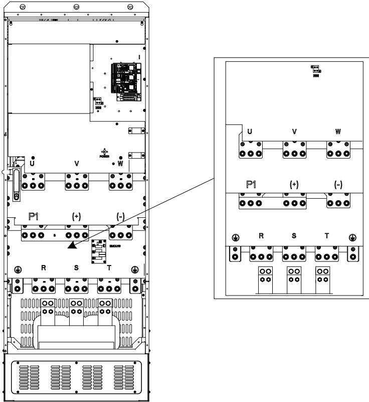
图 4-13 355G/400P~500G 主回路端子示意图
