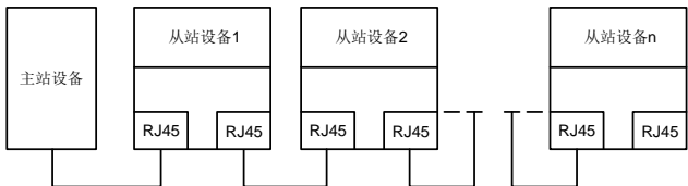
图 A-7 线型网络拓扑电气连接图
