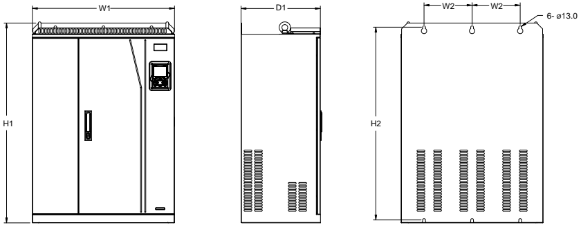
图 C-8 220G/250P~315G/350P 壁挂安装示意图
