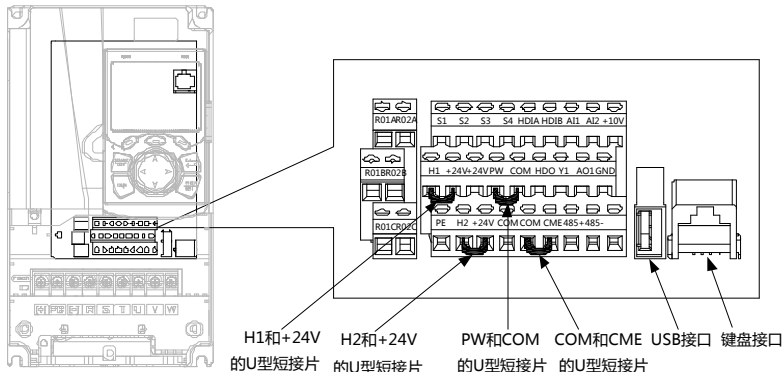
图 4-16 U 型短接位置示意图
