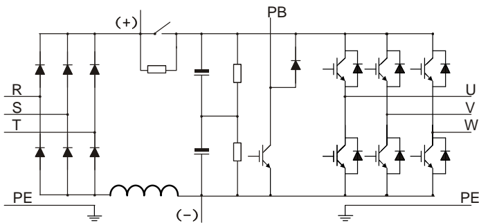
图 3-2 018G/022P~037G/045P 主回路简图
