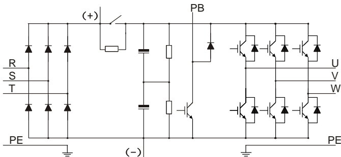
图 3-1 015G/018P 及以下主回路简图
