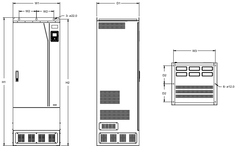
图 C-13 355G/400P~500G 落地安装示意图
