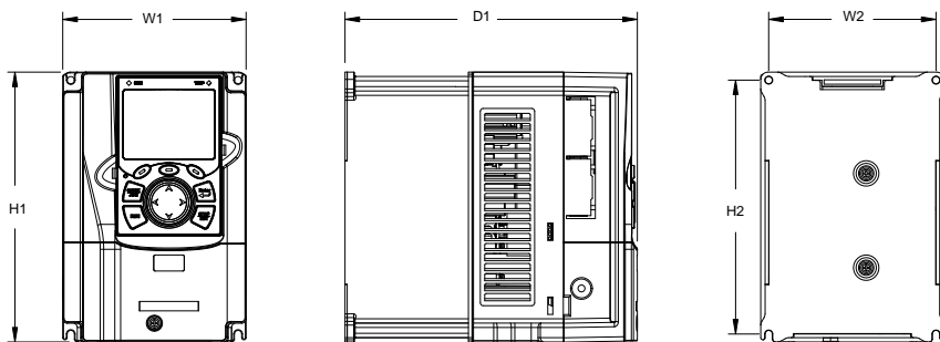
图 C-4 1R5G/2R2P~037G/045P 壁挂安装示意图
