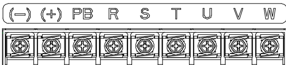
图 4-9 030G/037P-037G/045P 主回路端子示意图
