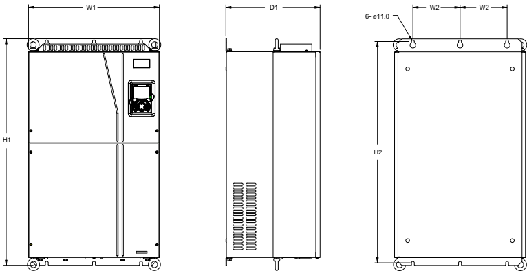
图 C-7 132G/160P~200G/220P 壁挂安装示意图
