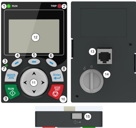
图 5-1 键盘示意图
