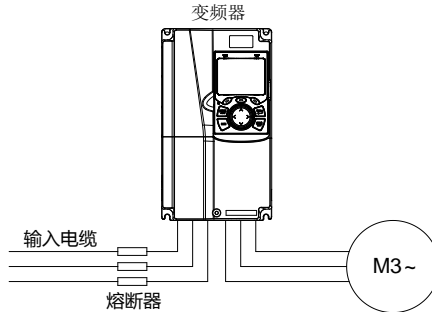
图 4-19 熔断器配置图
