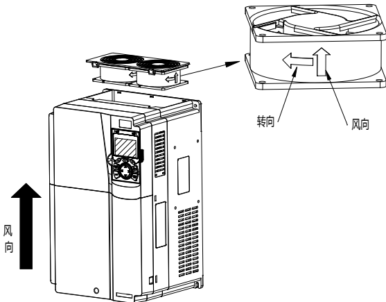
图 9-1 7R5G/011P (含) 以上机器风扇维护示意图
