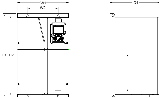
图 C-6 090G/110P~110G/132P 壁挂安装示意图
