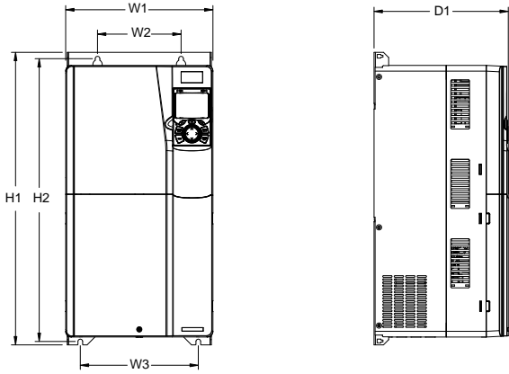
图 C-5 045G/055P~075G/090P 壁挂安装示意图
