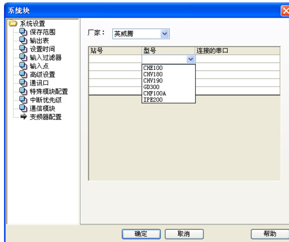
图2-13 变频器配置
