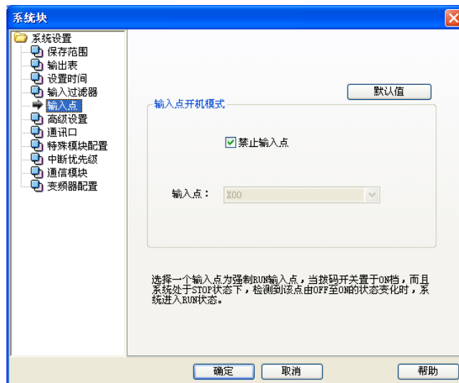
图2-7 设置输入点
