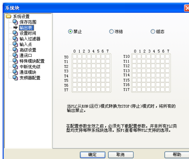
图2-4 设置输出表
