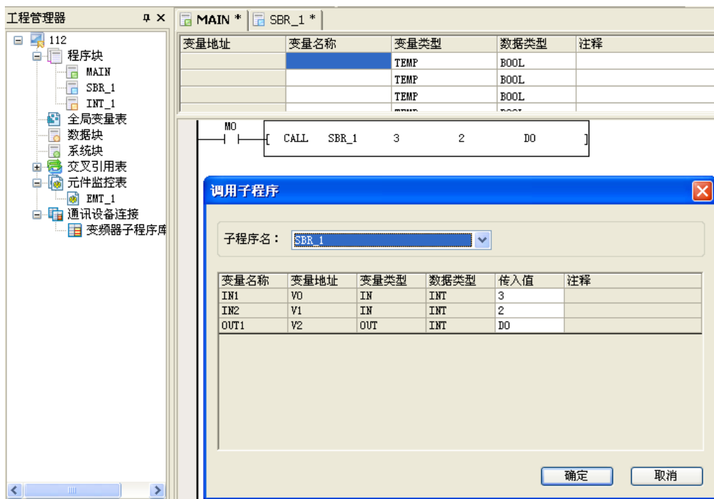
图4-12 调用子程序
