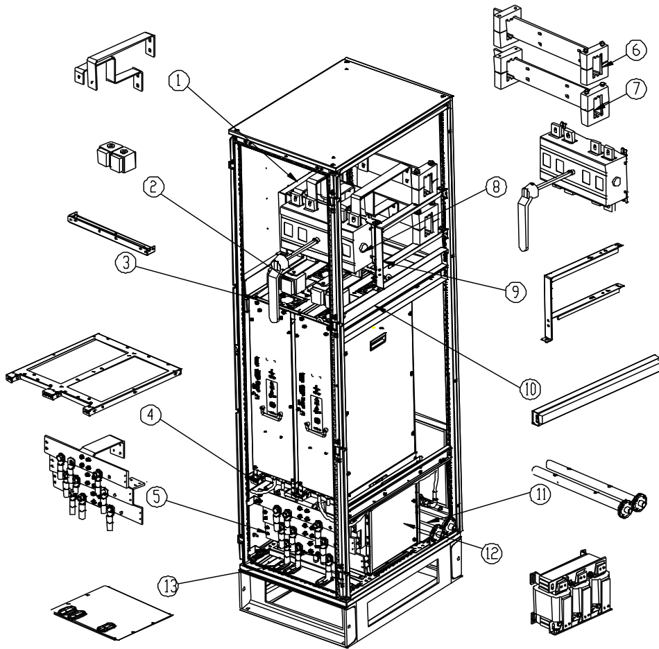
图 3-9 带隔离开关逆变柜 600mm 宽柜体安装示意图
