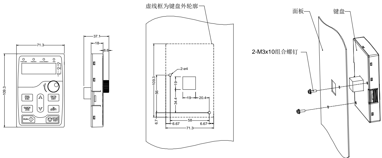
图 3-18 LED 键盘结构图
