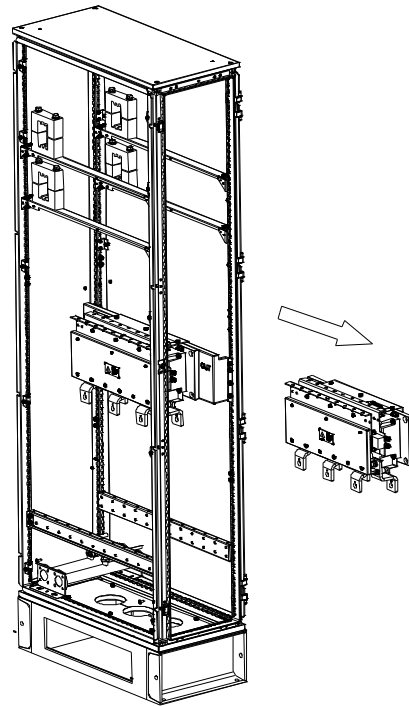
图 6-8 拆出水冷整流单元
