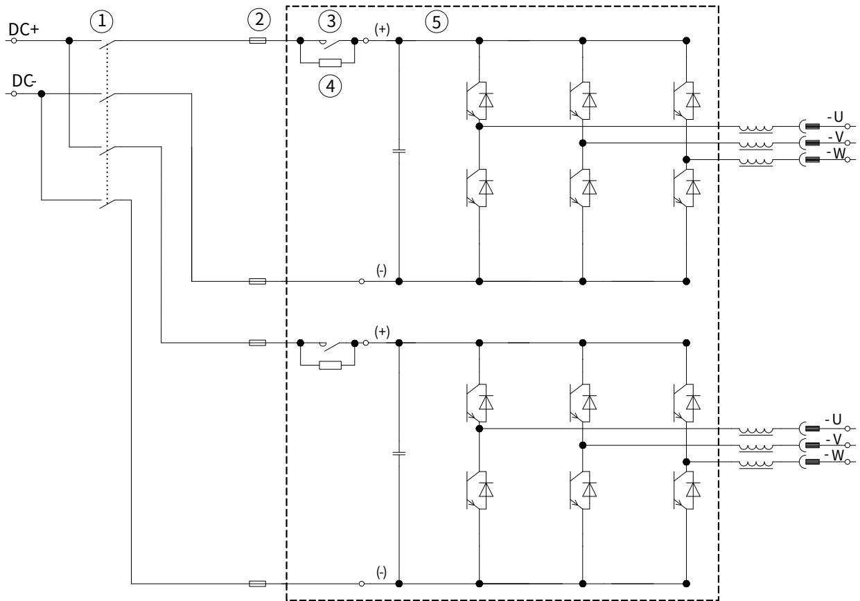
图 2-11 水冷逆变单元并机主回路简图
