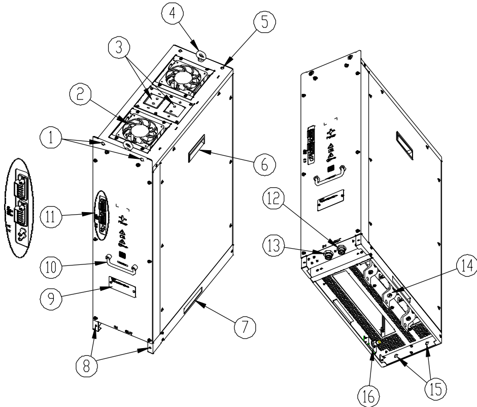
图 2-13 水冷逆变单元结构示意图
