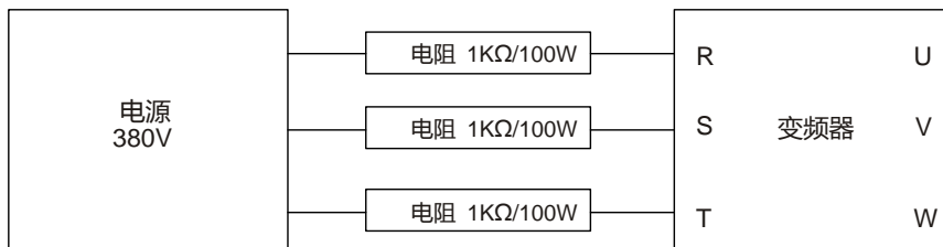
图 6-1 380V 驱动装置充电电路示例
