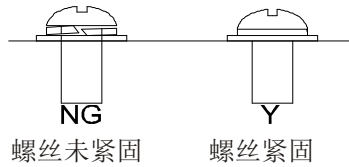
图 4-14 螺丝安装安装要求图
