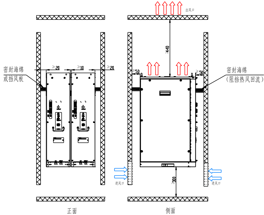
图 3-6 水冷变频及逆变单元对安装空间要求
