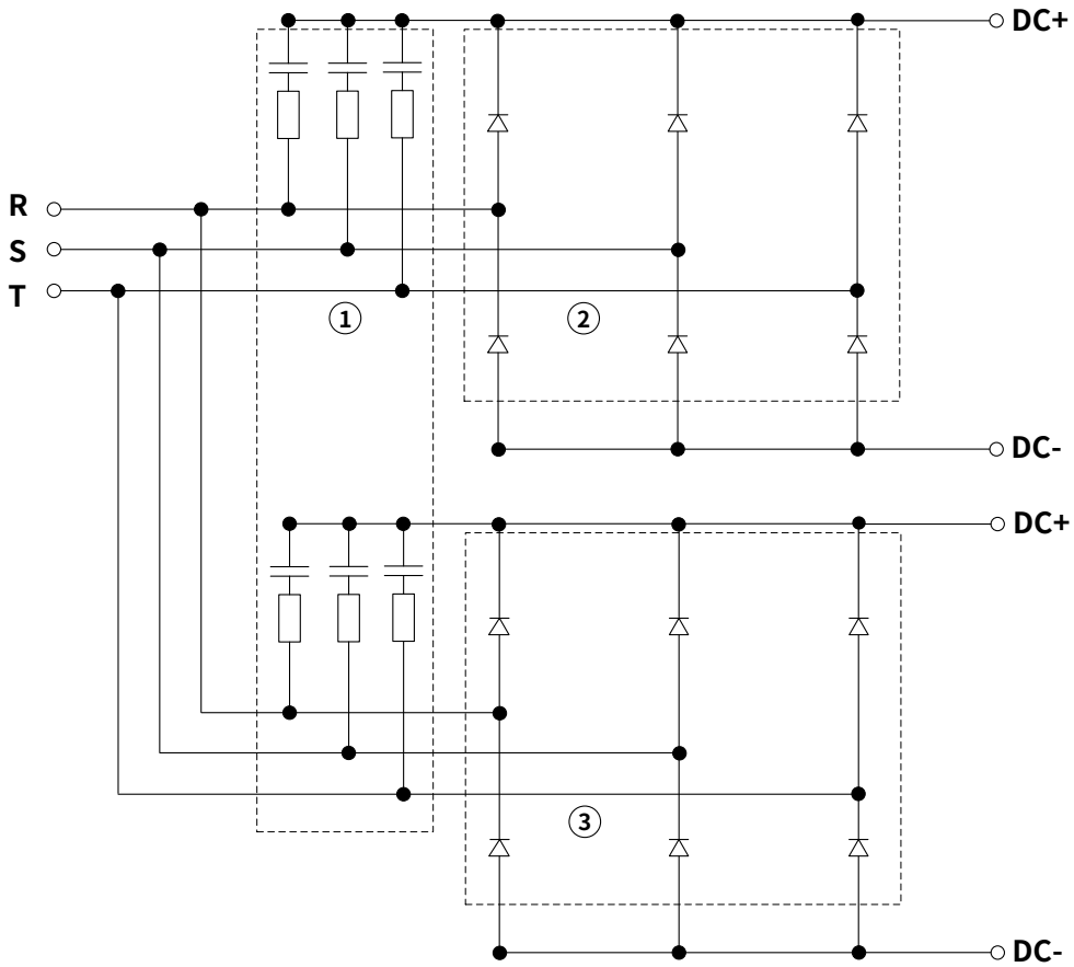
图 2-12 水冷整流单元
