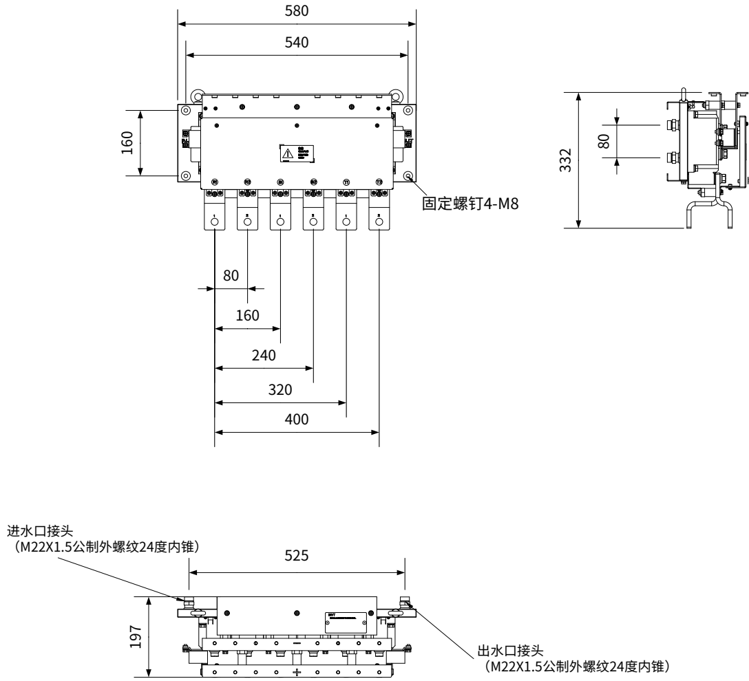
图 B-3 水冷变频器单元安装尺寸图
