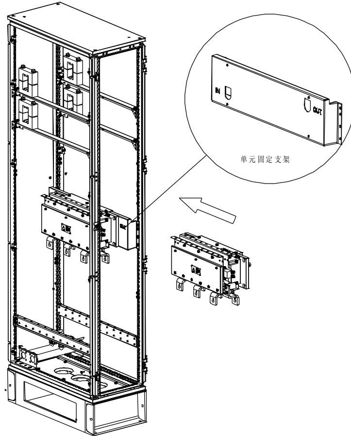
图 3-16 单元安装入柜示意图
