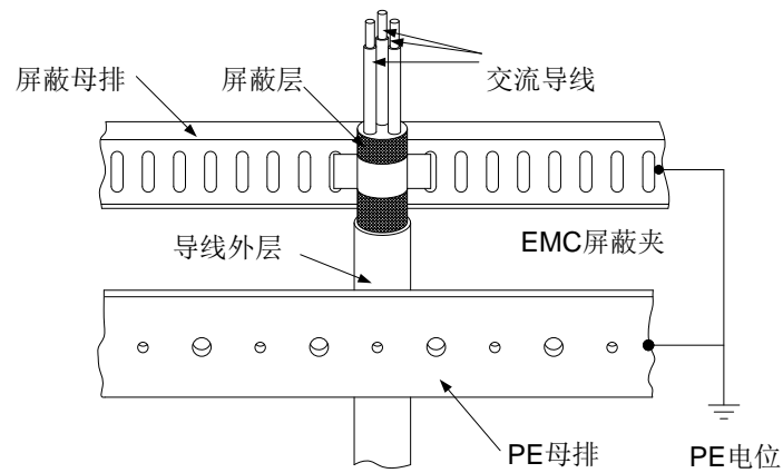
图 4-8 功率电缆屏蔽连接示意图
