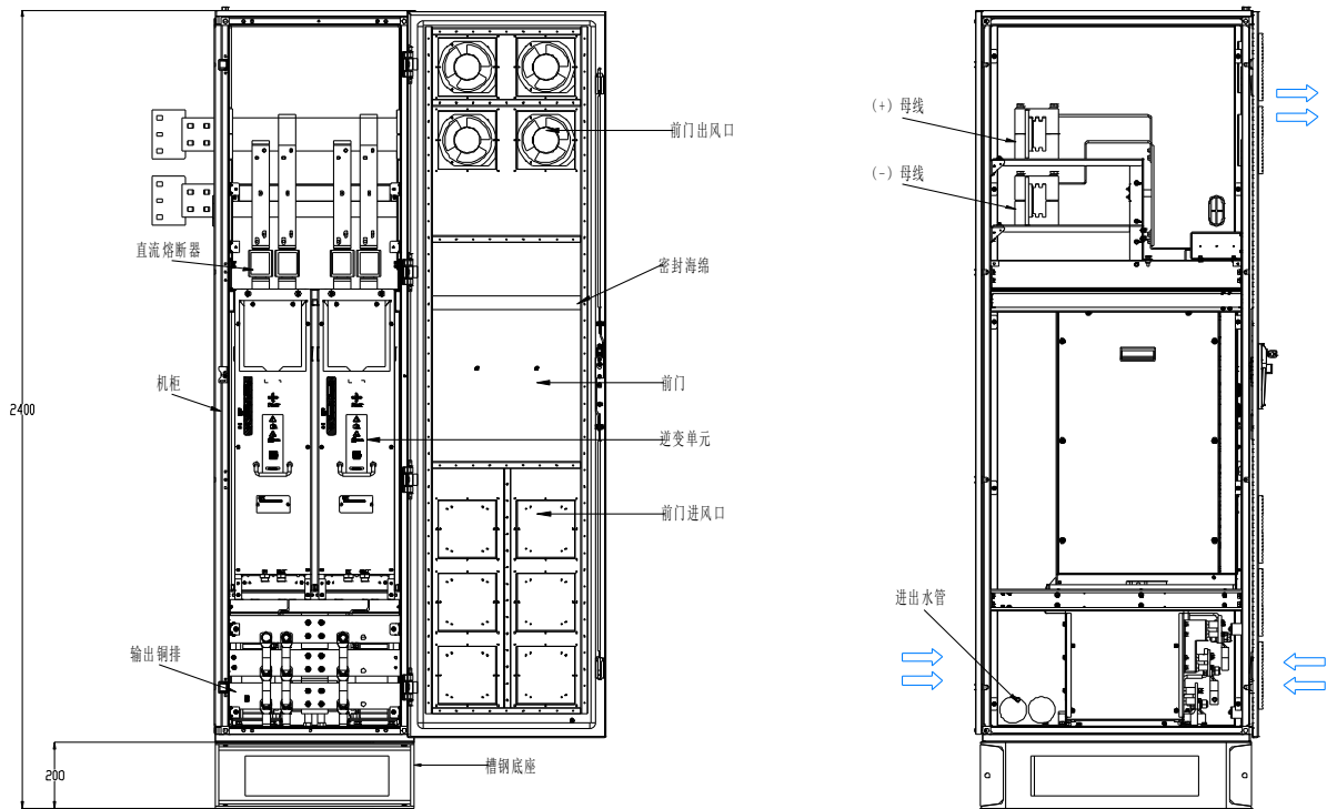
图 3-10 不带隔离开关逆变柜 600mm 宽柜体布局
