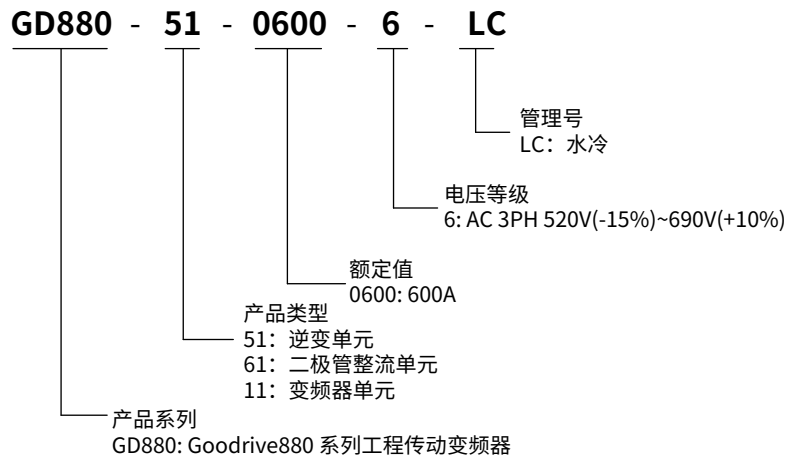
图 2-2 产品型号
