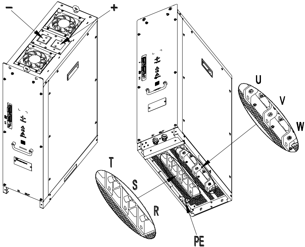
图 4-13 水冷变频器单元端子图
