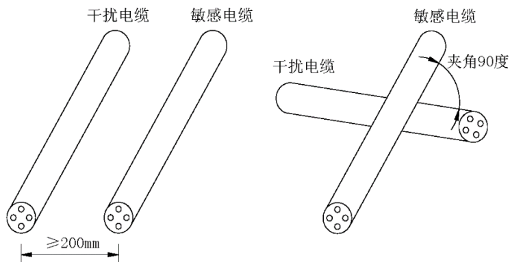
图 4-4 敏感电缆与干扰电缆布线示意图
