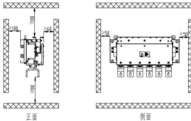
图 3-7 水冷整流单元对安装空间要求
