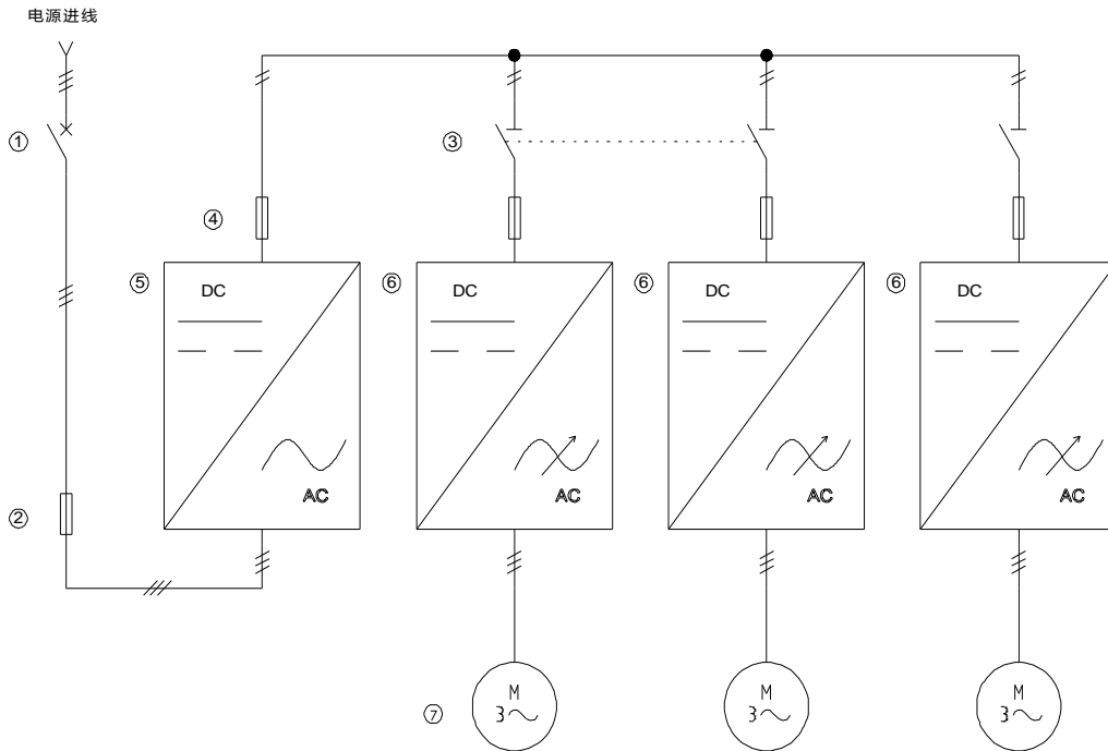
图 2-16 系统配置描述
