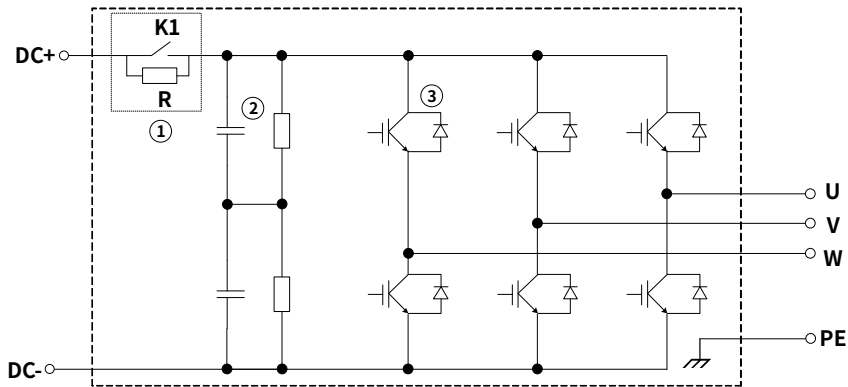
图 2-8 水冷逆变单元主回路简图
