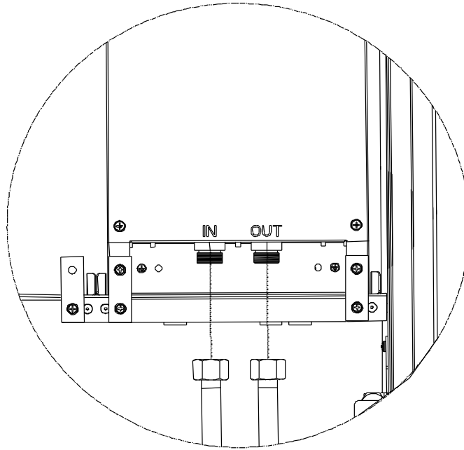
图 6-3 拆卸冷却管道
