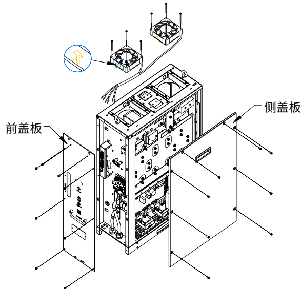
图 6-2 水冷逆变单元风扇维护示意图
