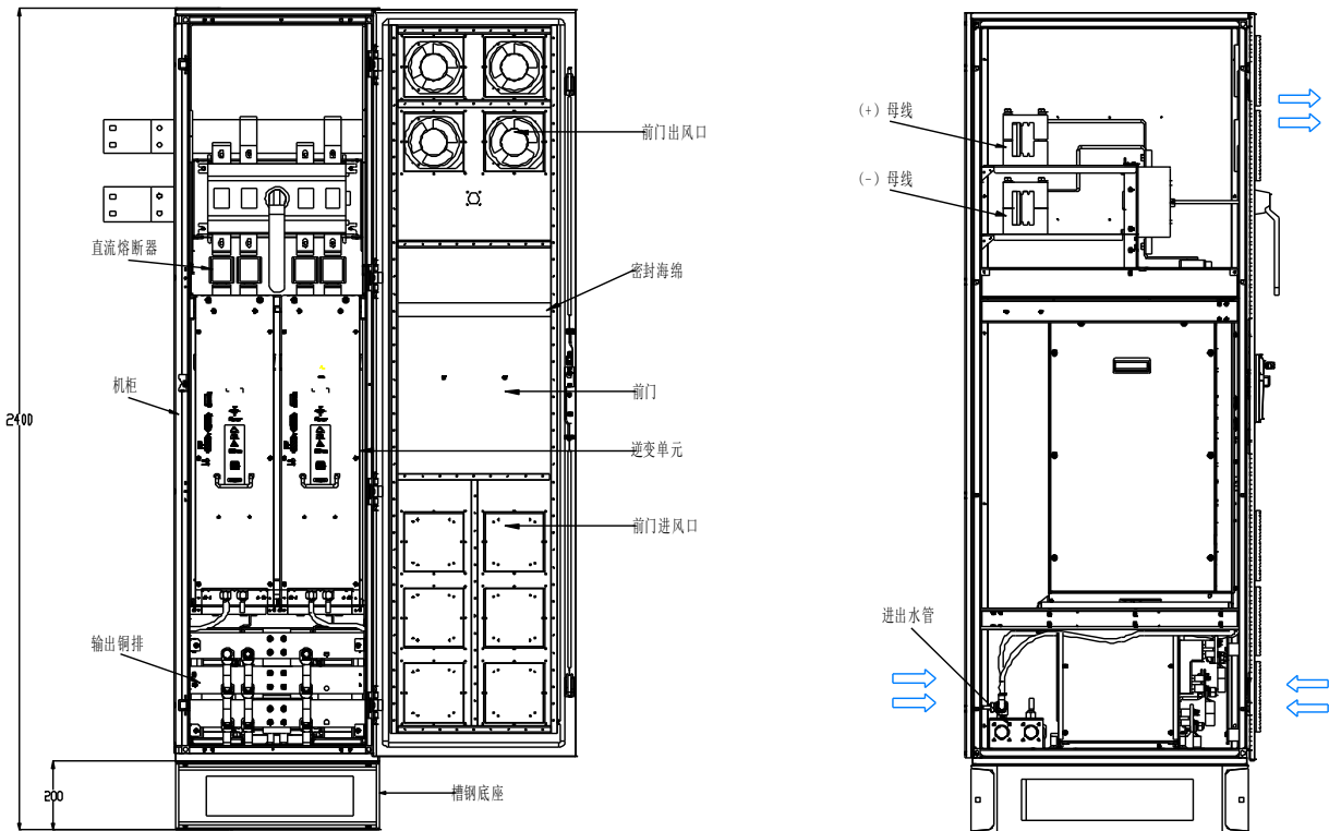
图 3-8 A8LC 带隔离开关水冷逆变单元柜柜体布局
