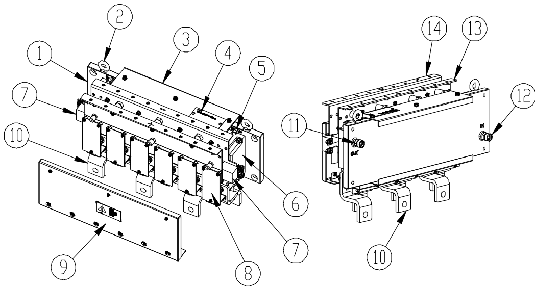
图 2-14 水冷整流单元结构示意图
