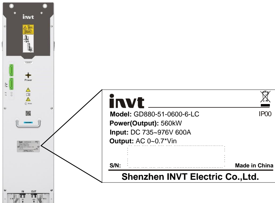
图 2-1 产品铭牌
