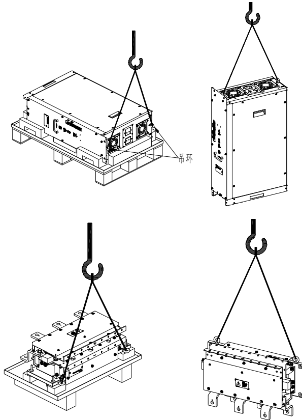
图 3-4 单元吊装示意图
