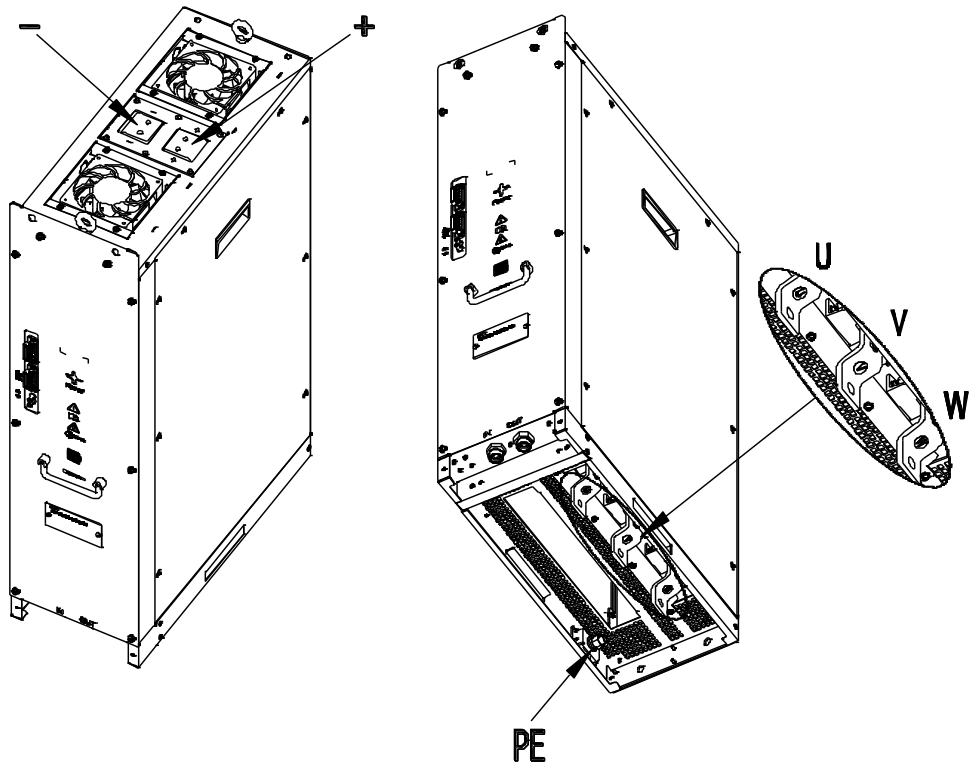
图 4-11 水冷逆变单元端子图
