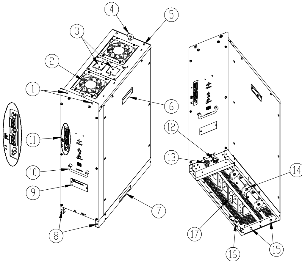
图 2-15 水冷变频器单元结构示意图
