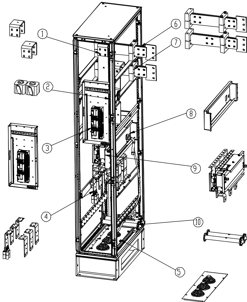
图 3-13 400mm 宽柜体安装示意图
