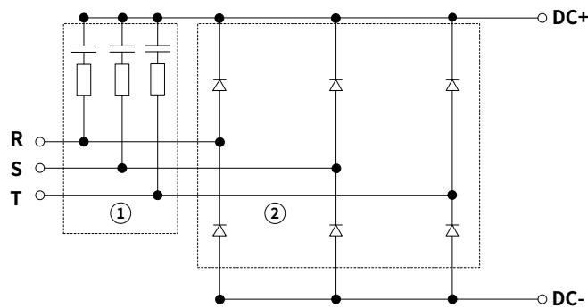
图 2-9 整流单元主回路简图
