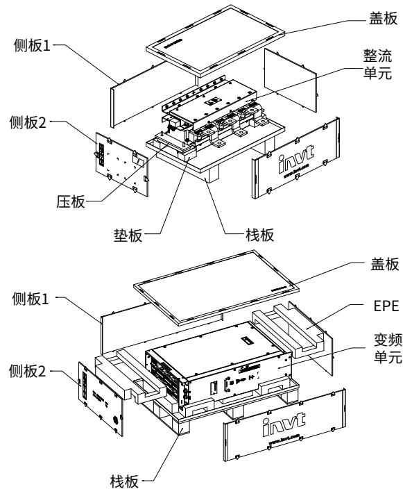
图 3-3 拆封示意图
