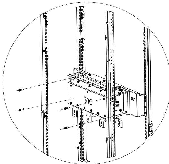
图 6-7 拆卸单元水冷板上 4 颗固定螺钉
