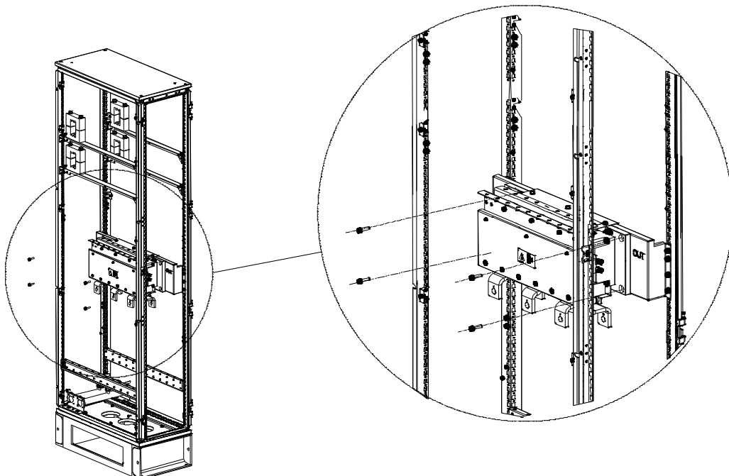
图 3-17 单元安装入柜示意图
