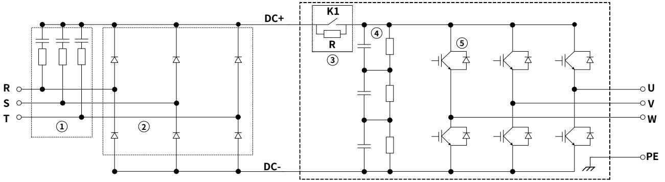
图 2-10 变频器单元主回路简图
