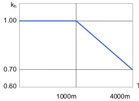
图 2-5 海拔高度降额
