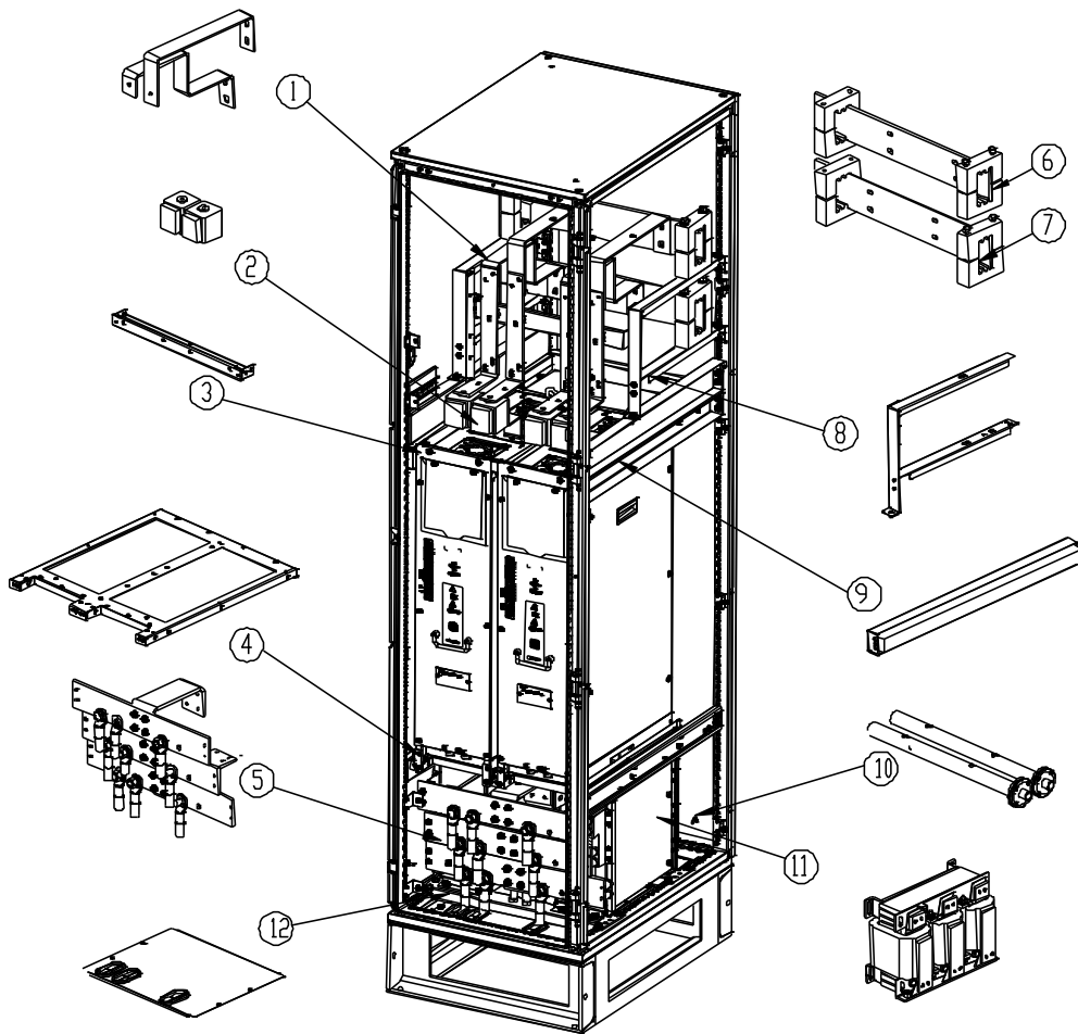
图 3-11 不带隔离开关逆变柜 600mm 宽柜体安装示意图
