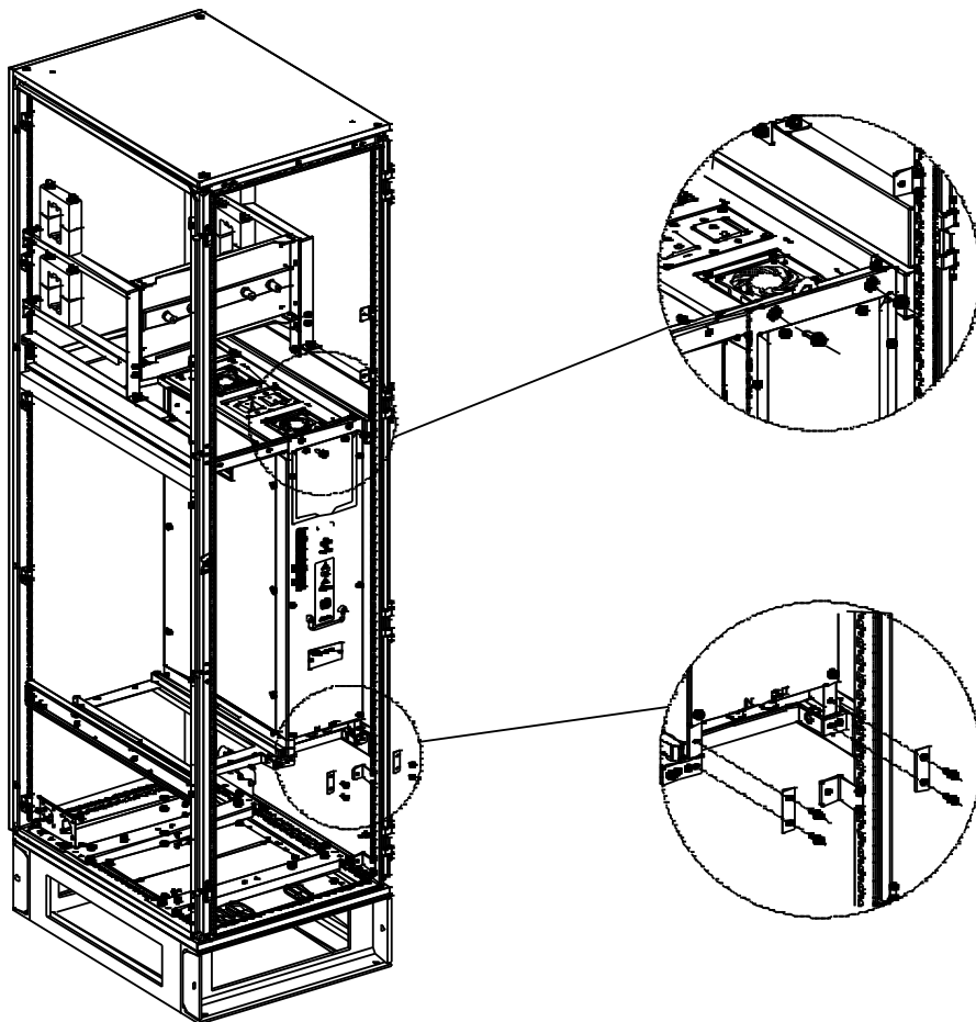
图 6-4 拆卸单元顶部和底部固定螺钉
