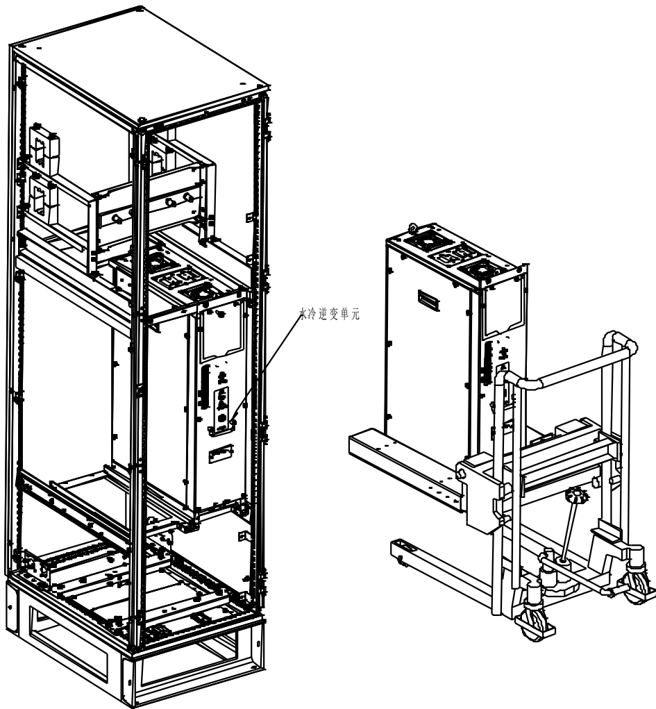
图 6-5 拉出水冷逆变单元
