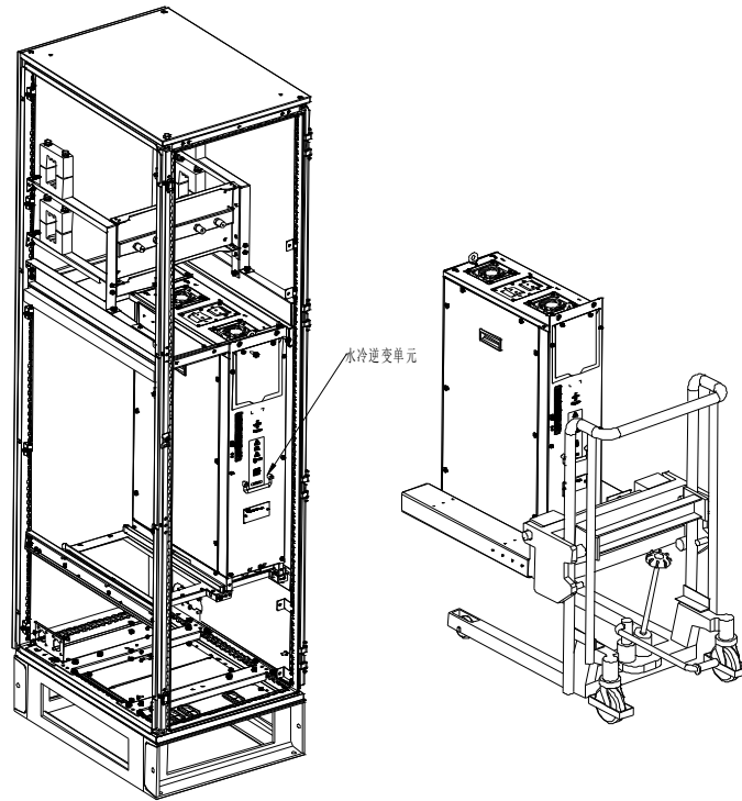
图 3-14 单元安装入柜示意图
