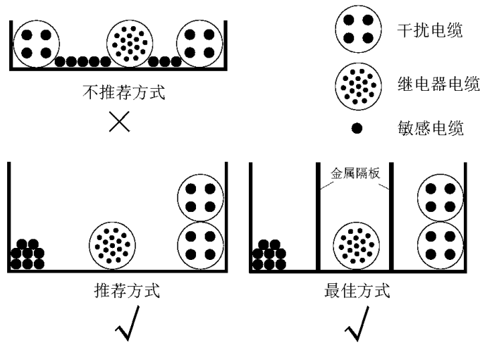
图 4-6 多种电缆敷设示意图
