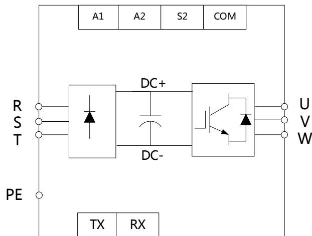
图 4-10 A8LC 变频器单元接线图
