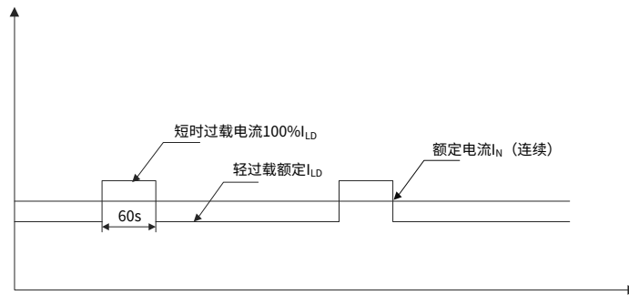
图 2-6 轻过载应用
