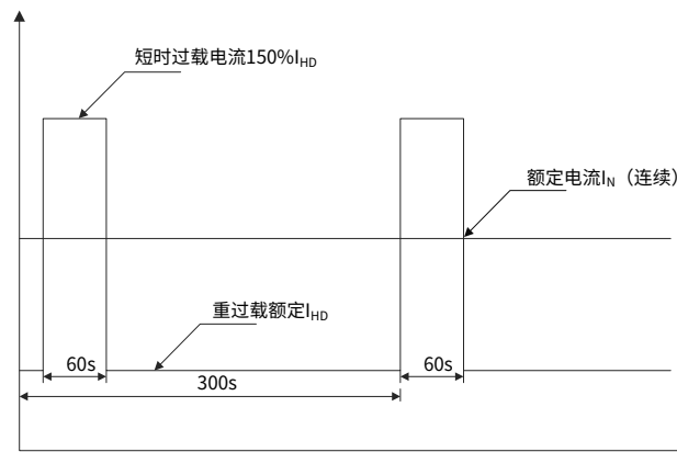
图 2-7 重过载应用
