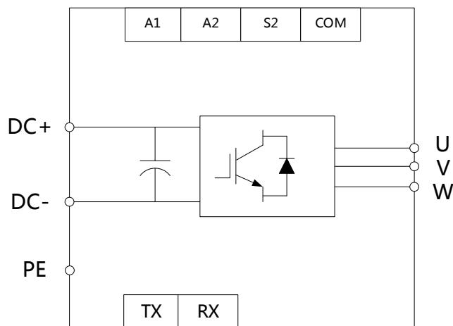
图 4-9 A8LC 逆变单元接线图
