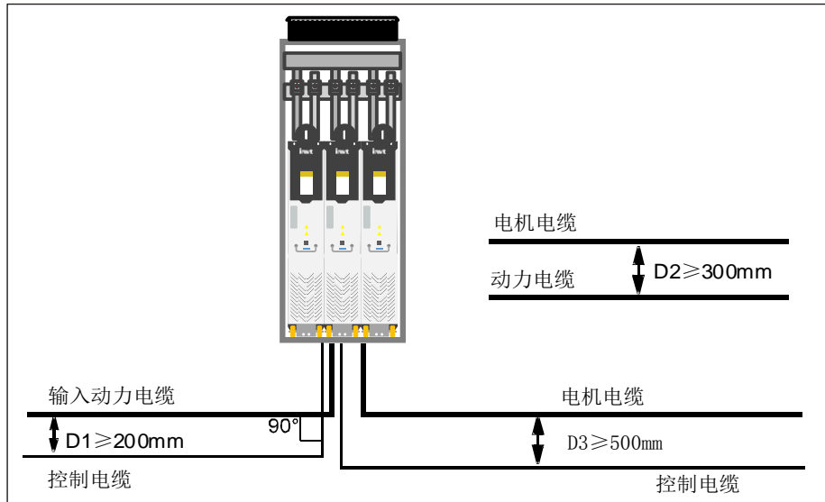
图 4-3 电缆布置一般原则
