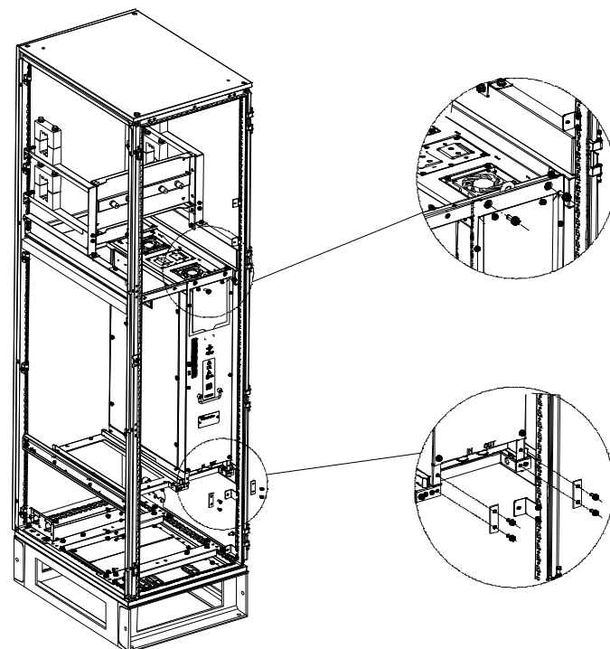
图 3-15 单元安装入柜示意图
