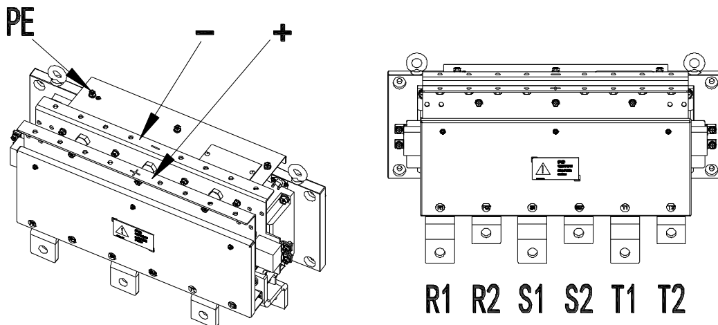
图 4-12 水冷整流单元端子图
