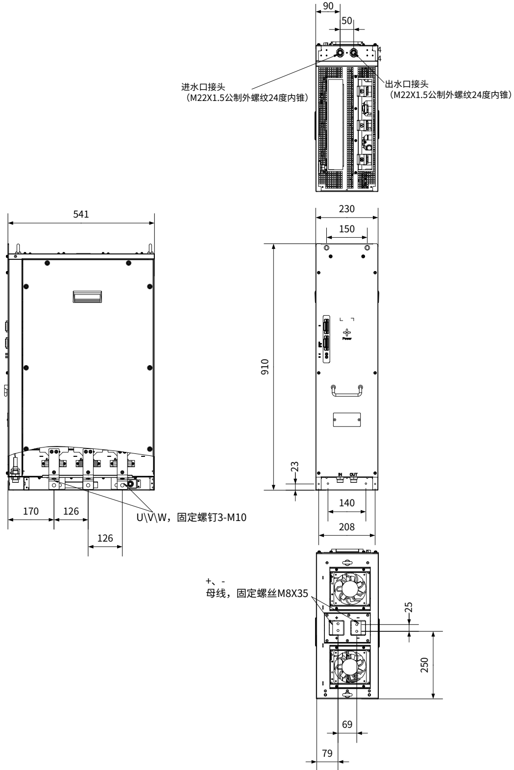
图 B-1 水冷逆变单元安装尺寸图
