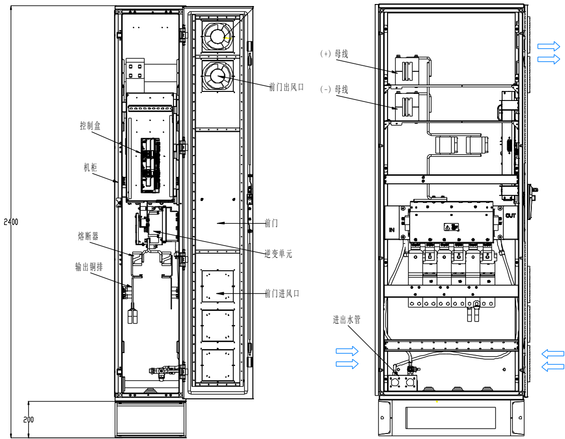
图 3-12 400mm 宽柜体布局
