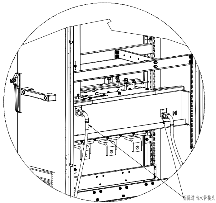
图 6-6 拆卸冷却管道
